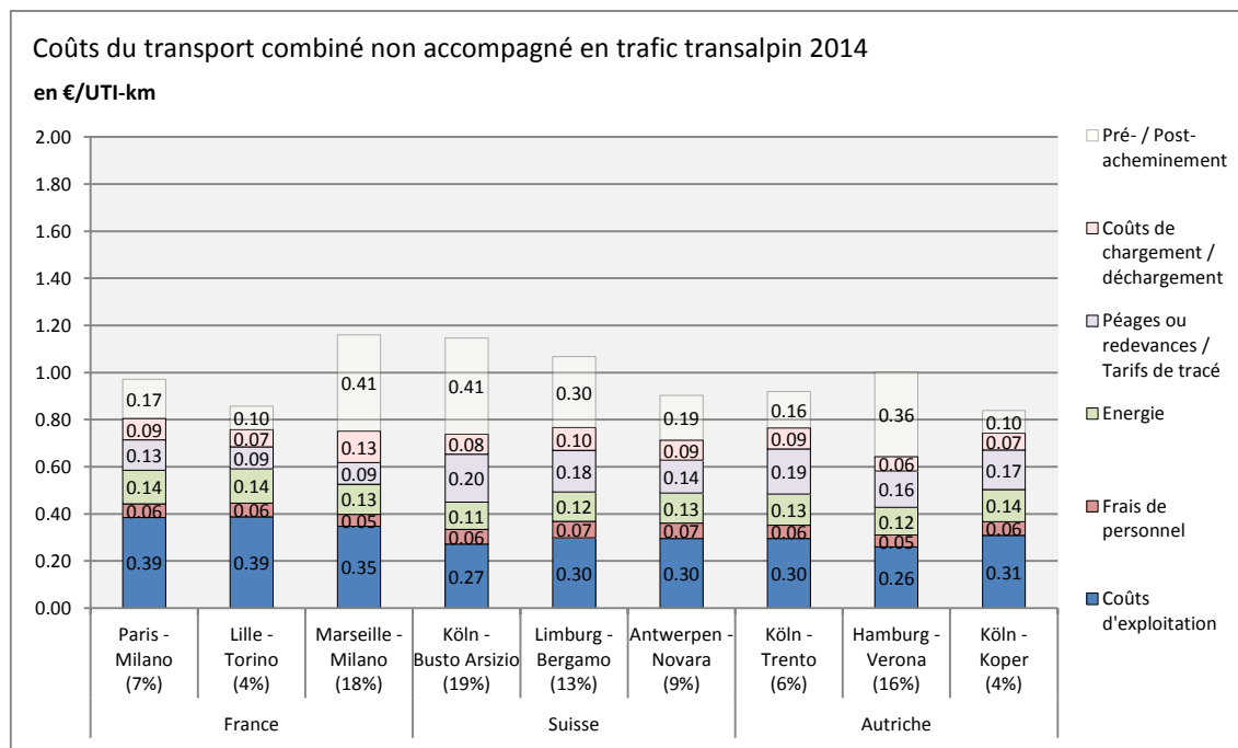
Figure 40: Coûts d'un transport combiné non accompagné en trafic transalpin 2014 (les valeurs en pourcentages représentent la partie route de la distance totale)
